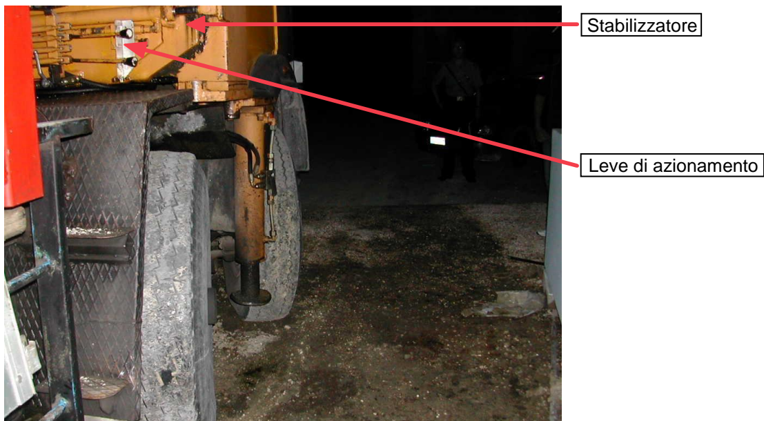
Figura 1. Autogrù al momento dell'infortunio con indicazione delle leve di azionamento e dello stabilizzatore
