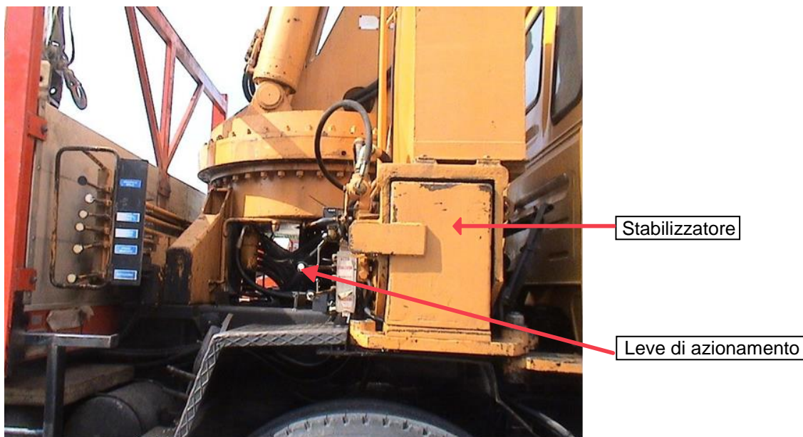
Figura 4. Autogrù con indicazione delle leve di azionamento e dello stabilizzatore
